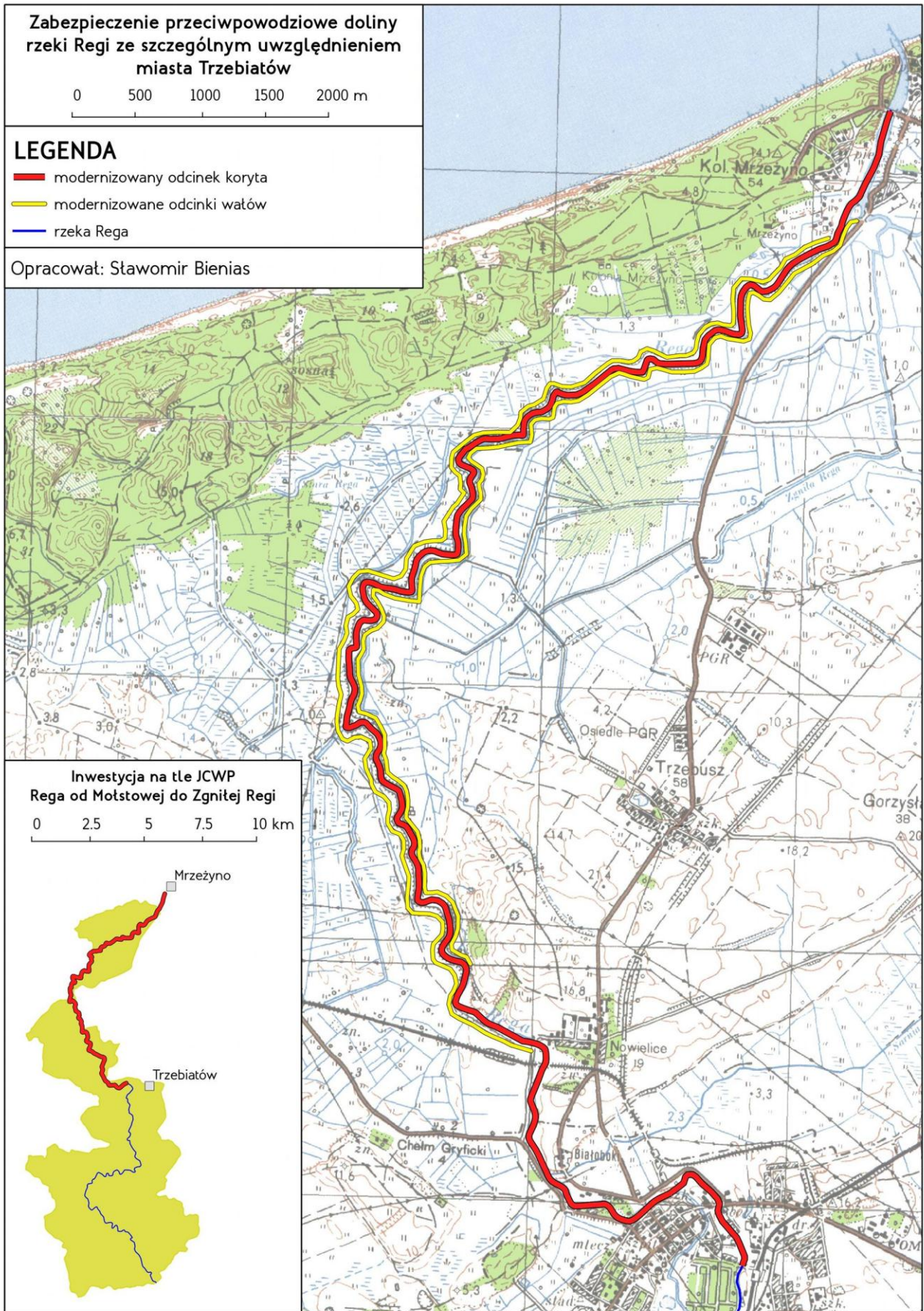
7. Zabezpieczenie przeciwpowodziowe doliny rzeki Regi ze szczególnym uwzględnieniem miasta Trzebiatów
