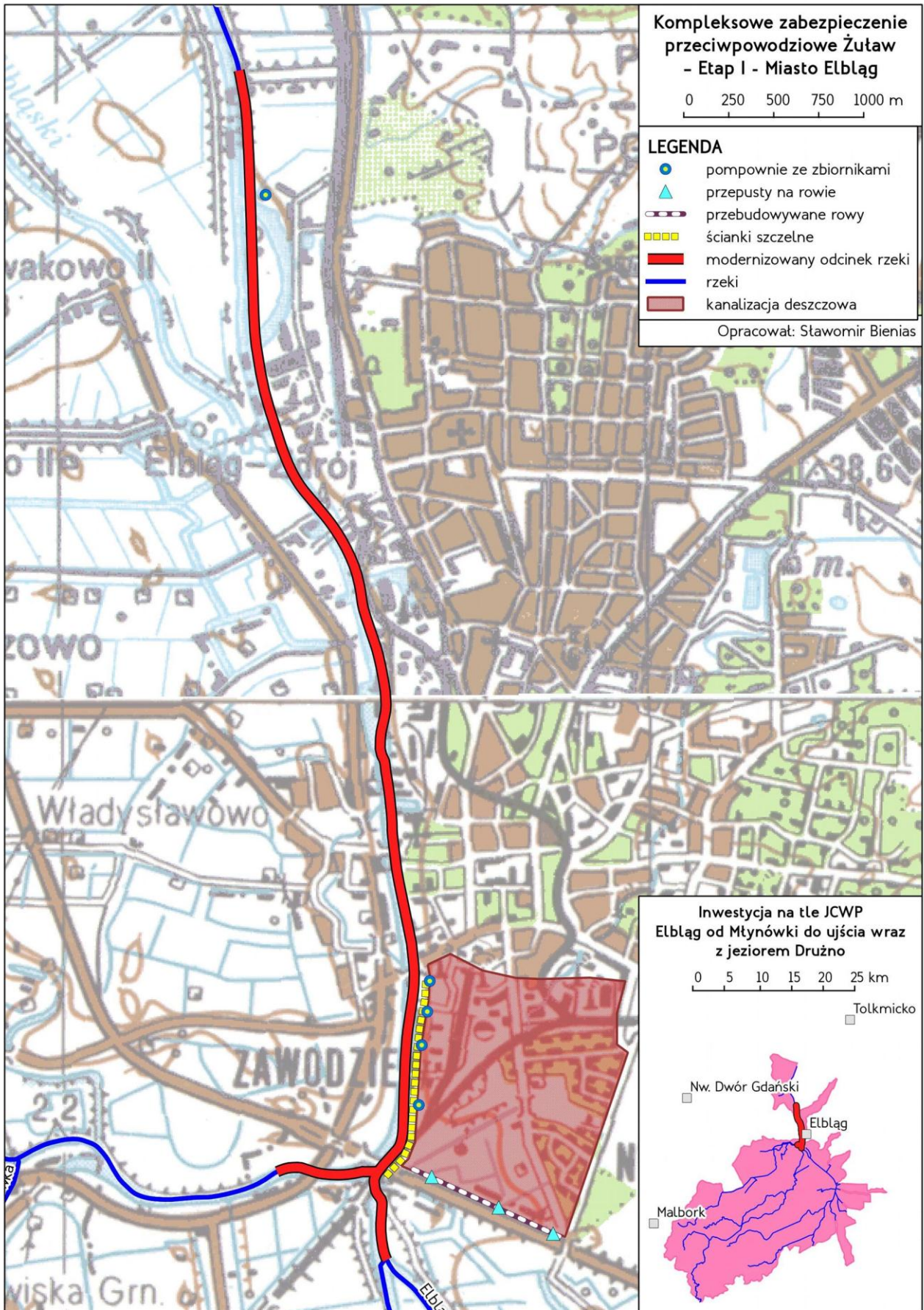
3. Kompleksowe zabezpieczenie przeciwpowodziowe Żuław – Etap I – Miasto Elbląg
