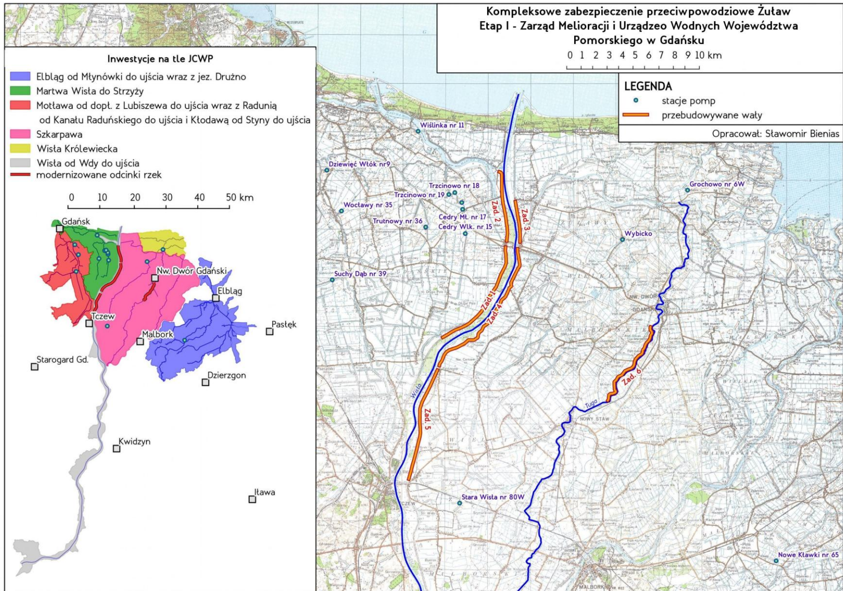
5. Kompleksowe zabezpieczenie przeciwpowodziowe Żuław – Etap I – Zarząd Melioracji i Urządzeń Wodnych w Gdańsku
