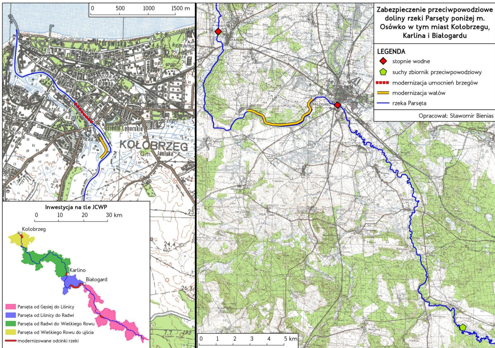
6. Zabezpieczenie przeciwpowodziowe doliny rzeki Parsęty poniżej m. Osówko w tym miast Kołobrzegu, Karlina i Białogardu
