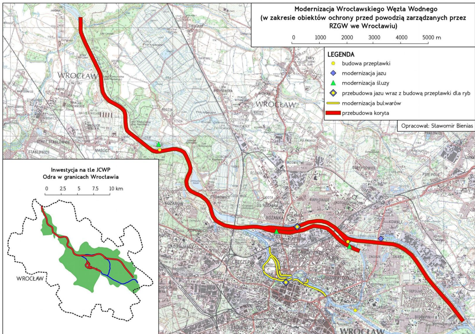
9. Modernizacja Wrocławskiego Węzła Wodnego (w zakresie obiektów ochrony przed powodzią zarządzanych przez RZGW we Wrocławiu)
