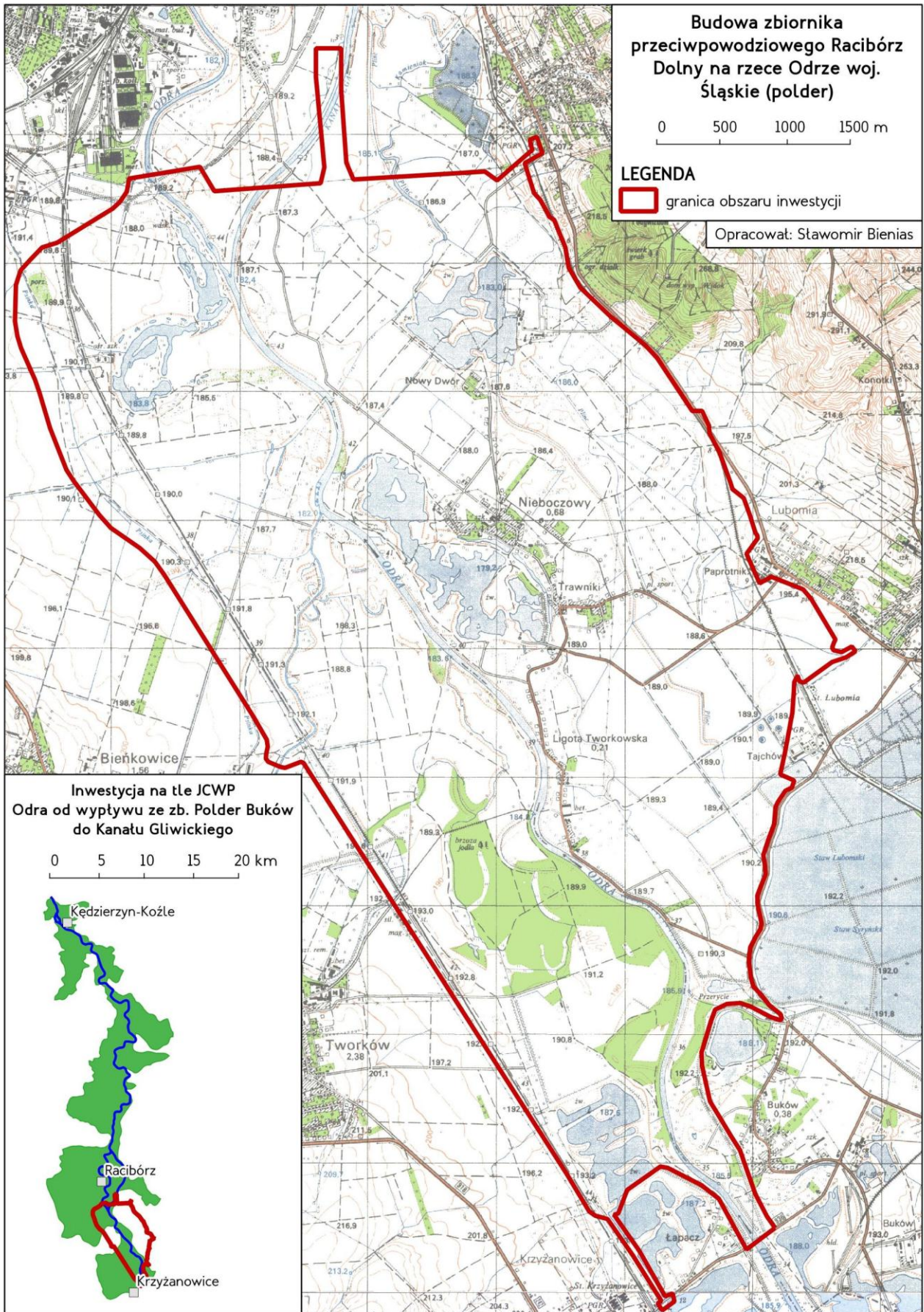
11. Budowa zbiornika przeciwpowodziowego Racibórz Dolny na rzece Odrze woj. śląskie (polder)
