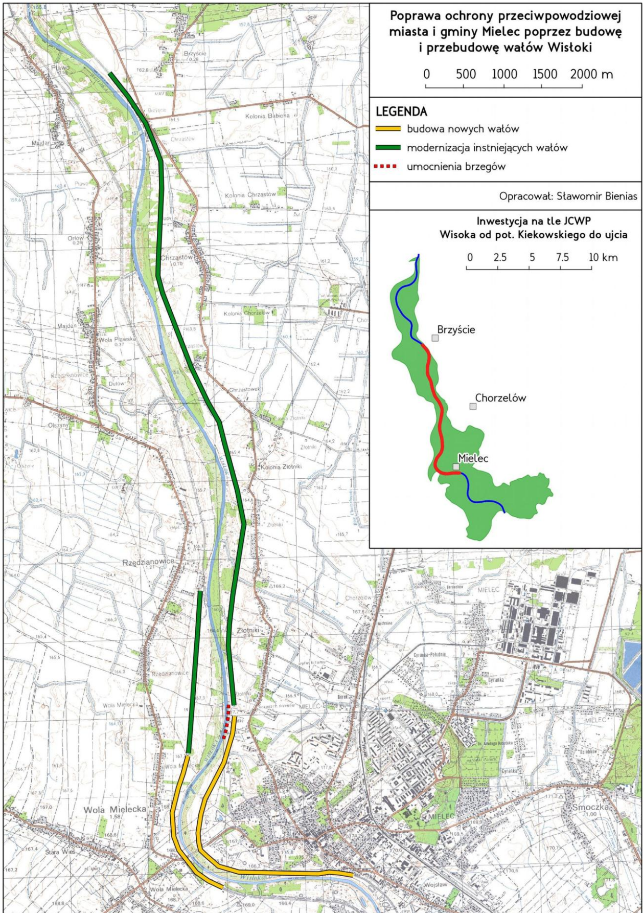
14. Poprawa stanu ochrony przeciwpowodziowej miasta i gminy Mielec poprzez budowę i przebudowę wałów Wisłoki
