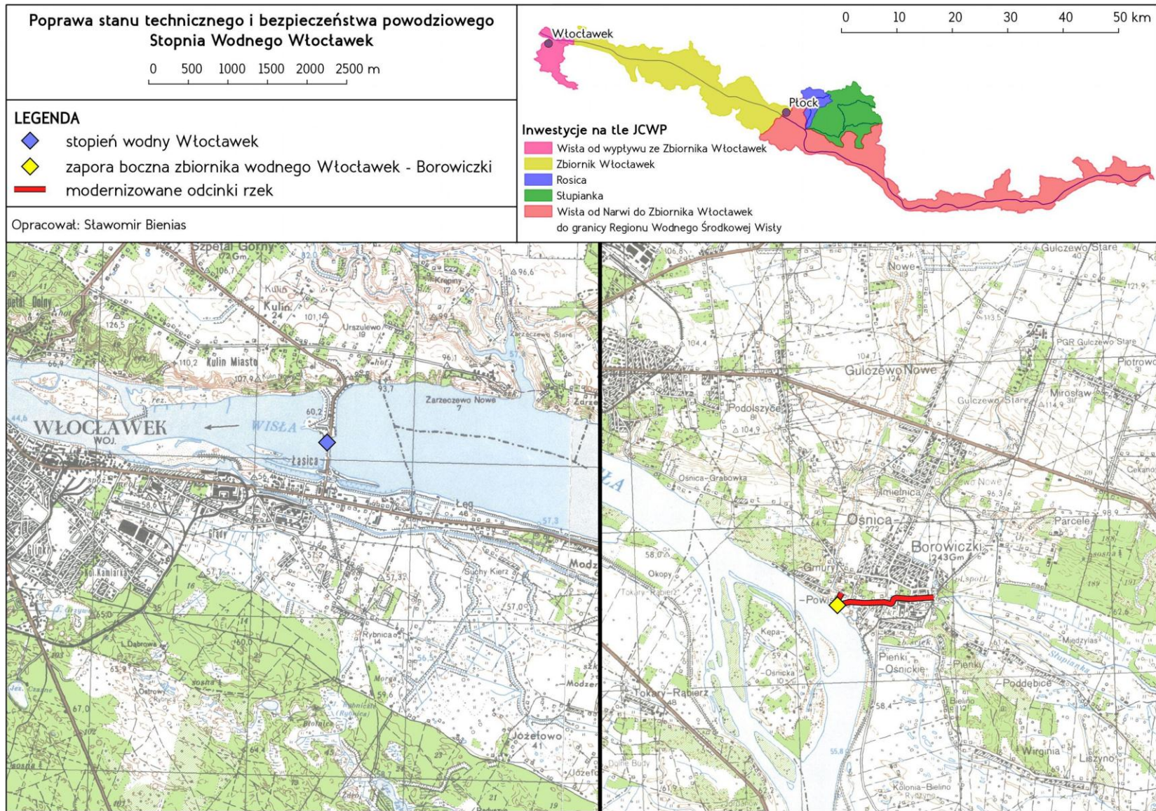
8. Poprawa stanu technicznego i bezpieczeństwa powodziowego Stopnia Wodnego Włocławek
