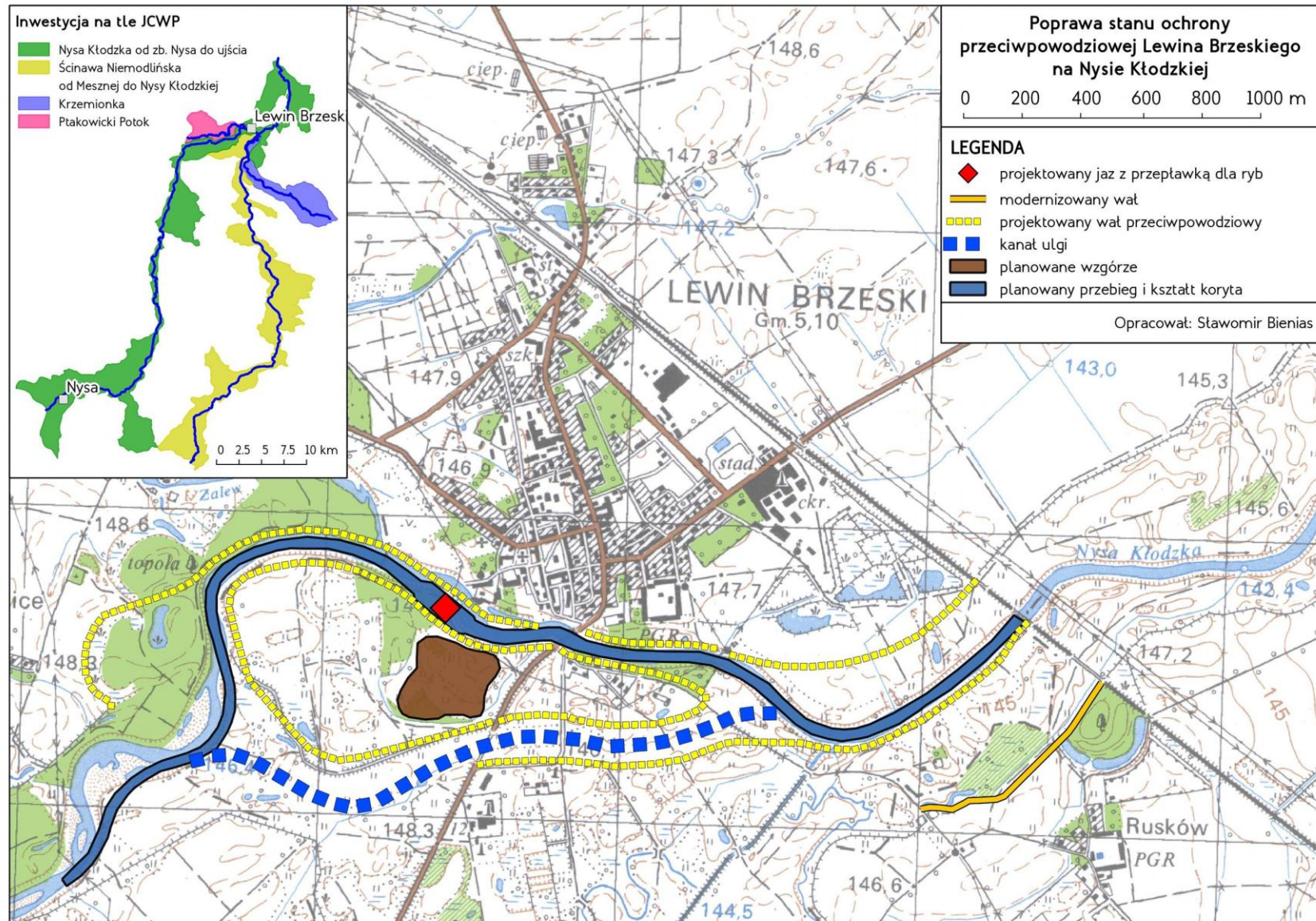
13. Poprawa stanu ochrony przeciwpowodziowej Lewina Brzeskiego na Nysie Kłodzkiej
