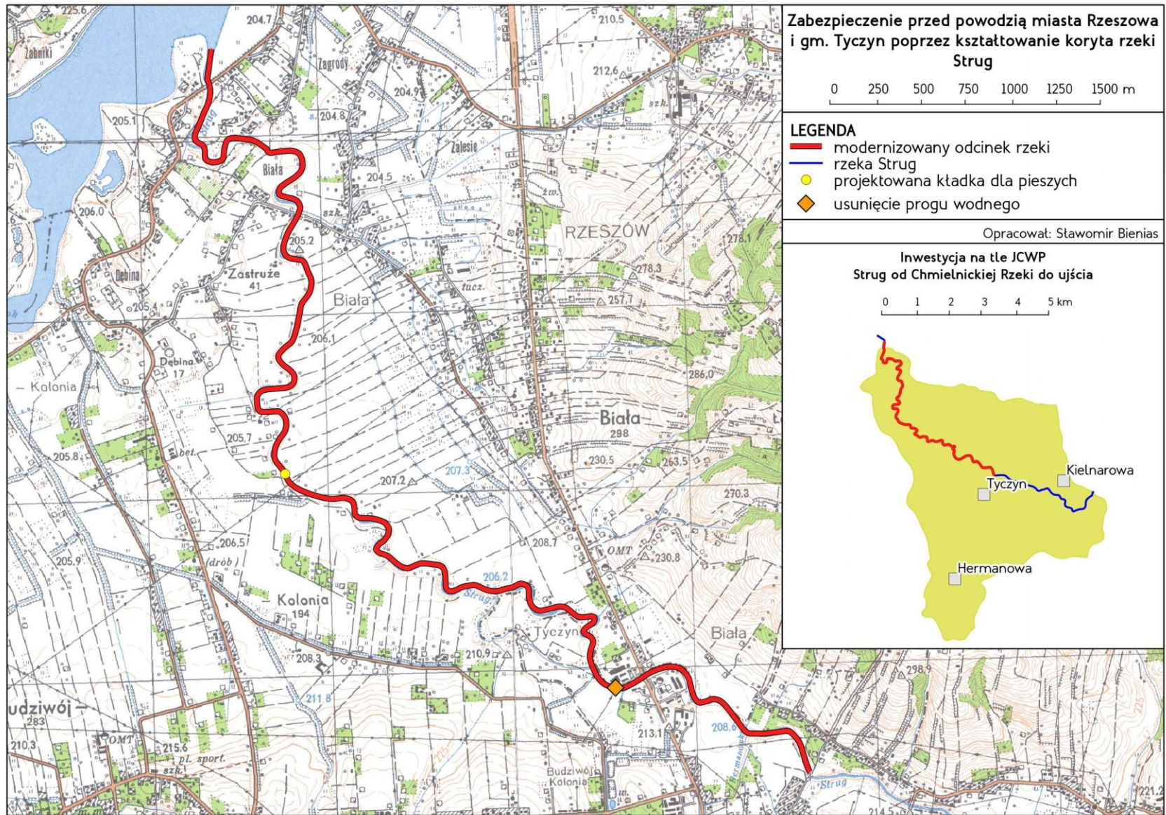
15. Zabezpieczenie przed powodzią miasta Rzeszowa i gm. Tyczyn przez kształtowanie koryta rzeki Strug
